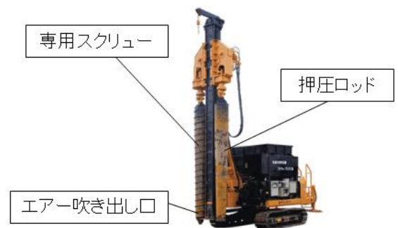
図-1 スクリー・プレス施工機
